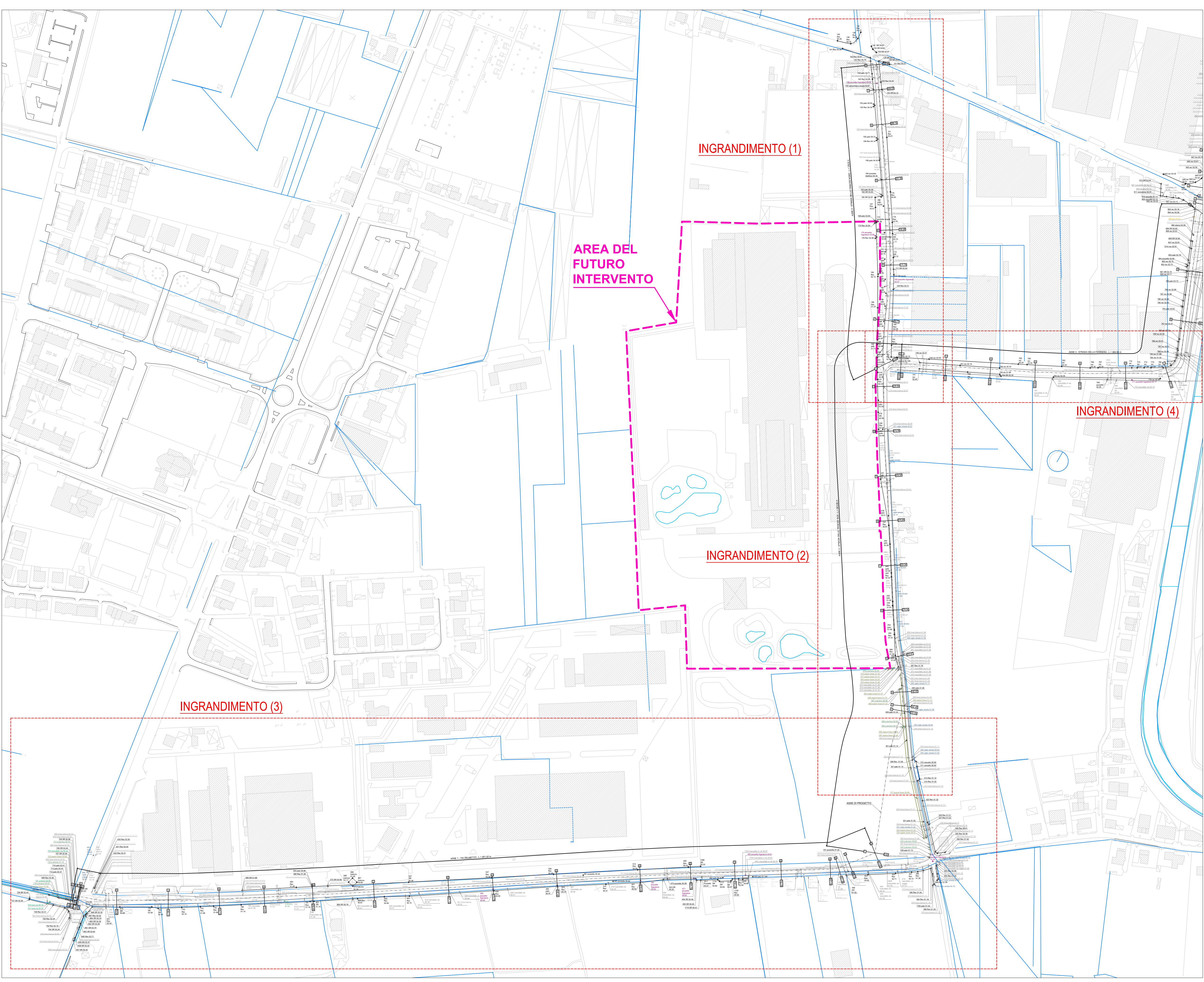
PLANIMETRIA DI INQUADRAMENTO Scala 1:2000
